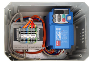
contrôleur / régulateur de débit
